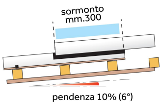
pendenza 10% (6°)
