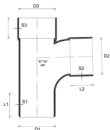
TS87 * DERIVAZIONE RACCORDATA
