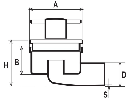
scarico orizzontale orientabile
