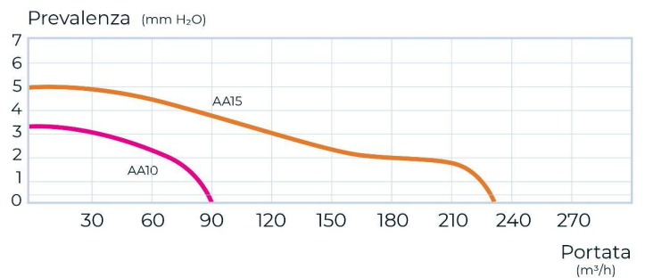
Curve di portata:
